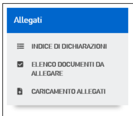
Figura 25 - Menu "Allegati"
